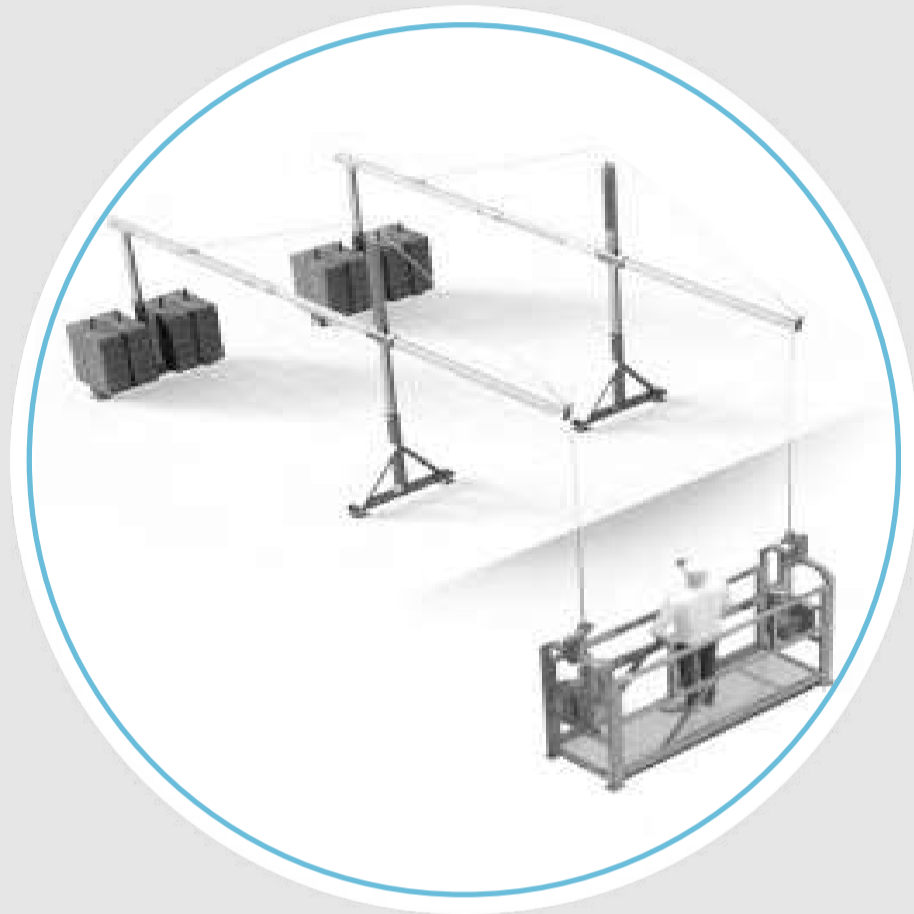
Telescópico rectangular contrapesado
