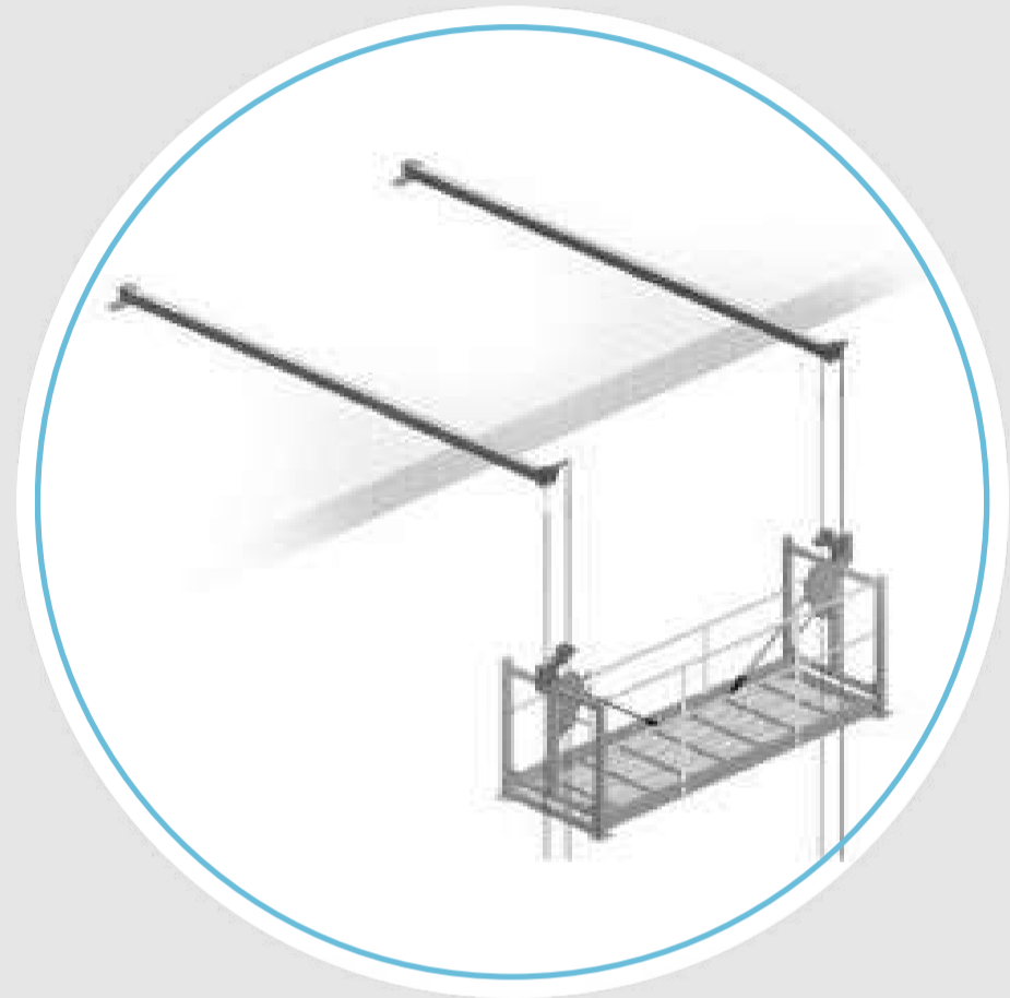
Anclaje a la losa de posición baja
