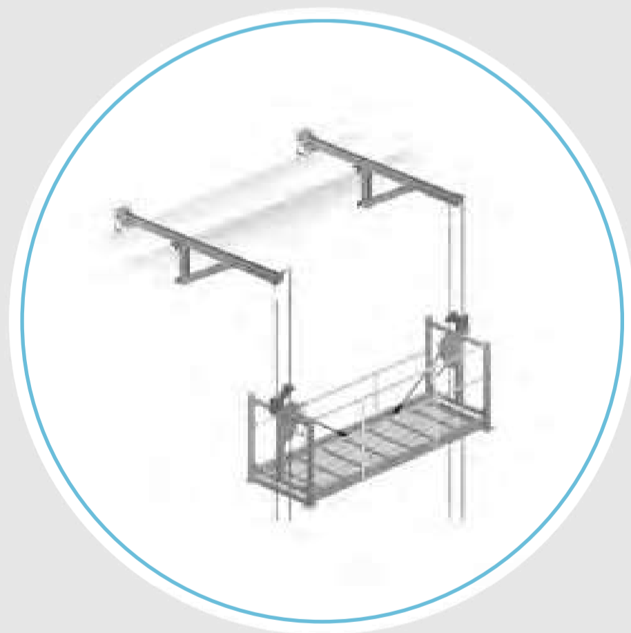
Pescante de antepecho tipo Clamp
